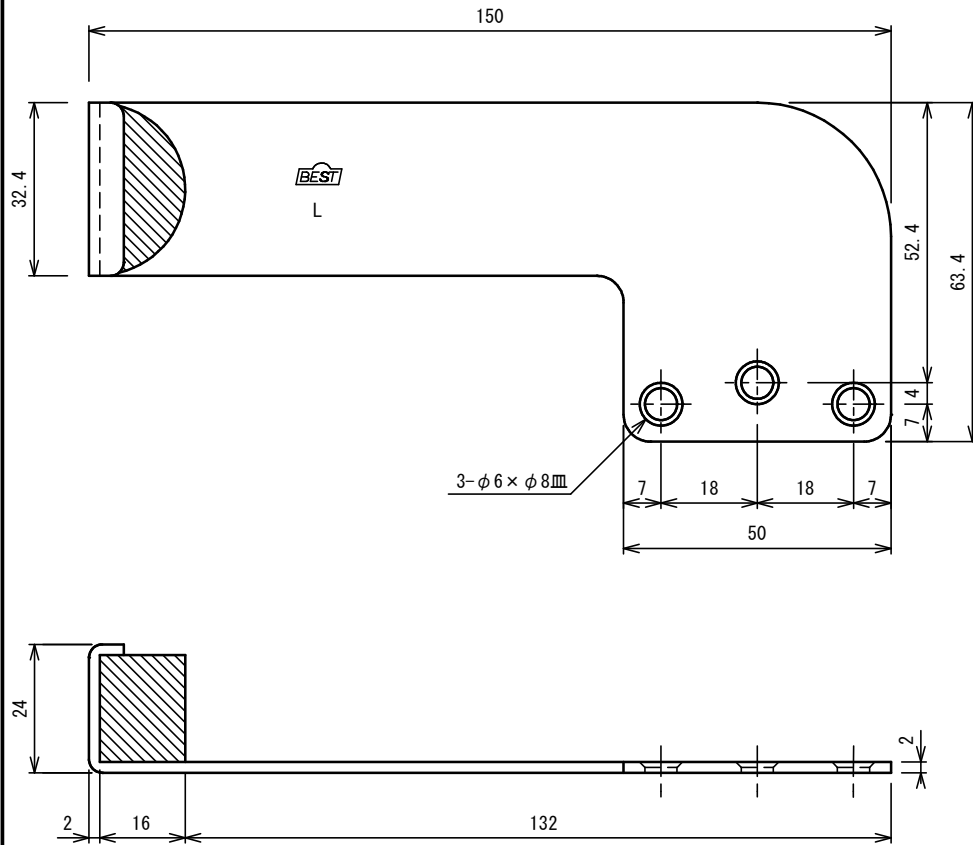
左勝手
