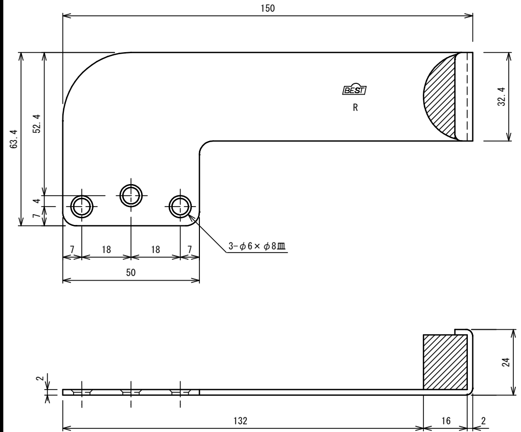
右勝手
