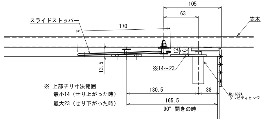
納まり図 (S=1/2)
