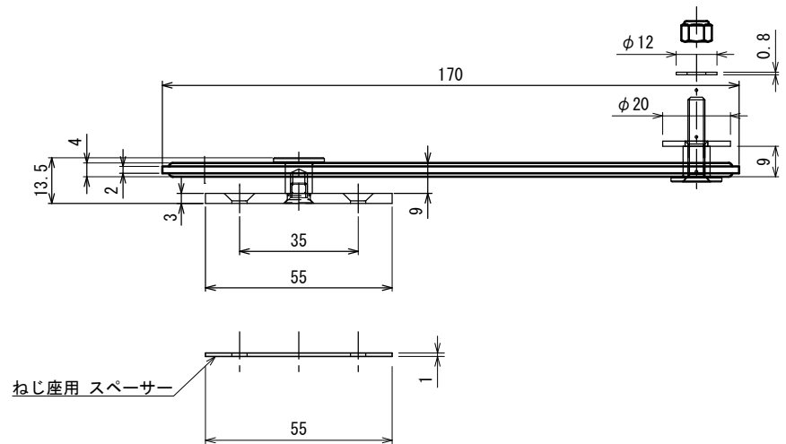
製品図 (S=1/1)
