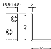
No.558-1・No.558-2 ※( )内はNo.558-2寸法
