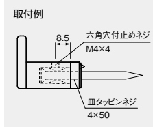
BA-707W (ダブル)
