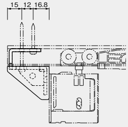
上吊レール 組合同
