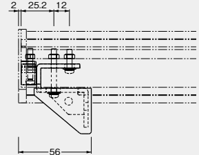
アウトセットレール・アウトセット用キャップ 組合同
