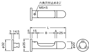
寸法表 (mm)
